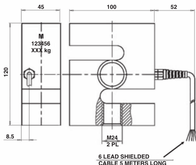
3000, 5000kg cell outline
